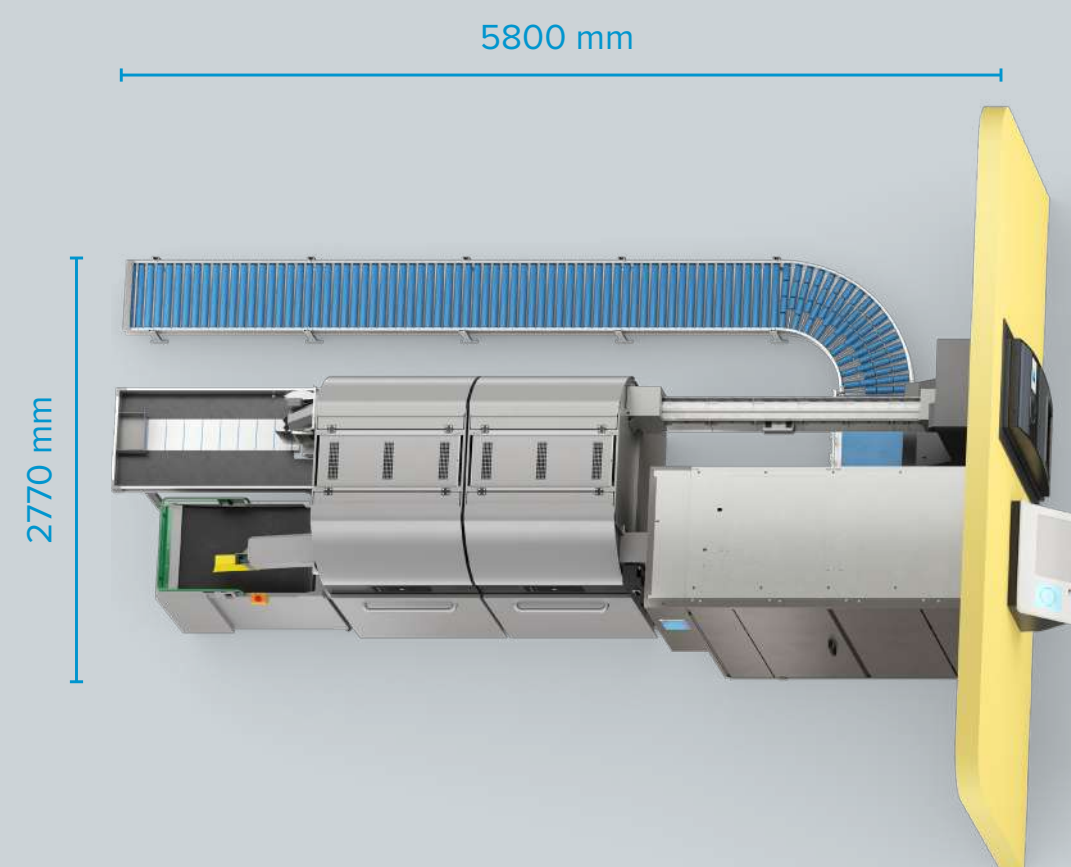
TOMRA R2+T9 z modułem MultiPac, stołem na butelki zwrotne, taśmą do transportu skrzynek i systemem SoftDrop
