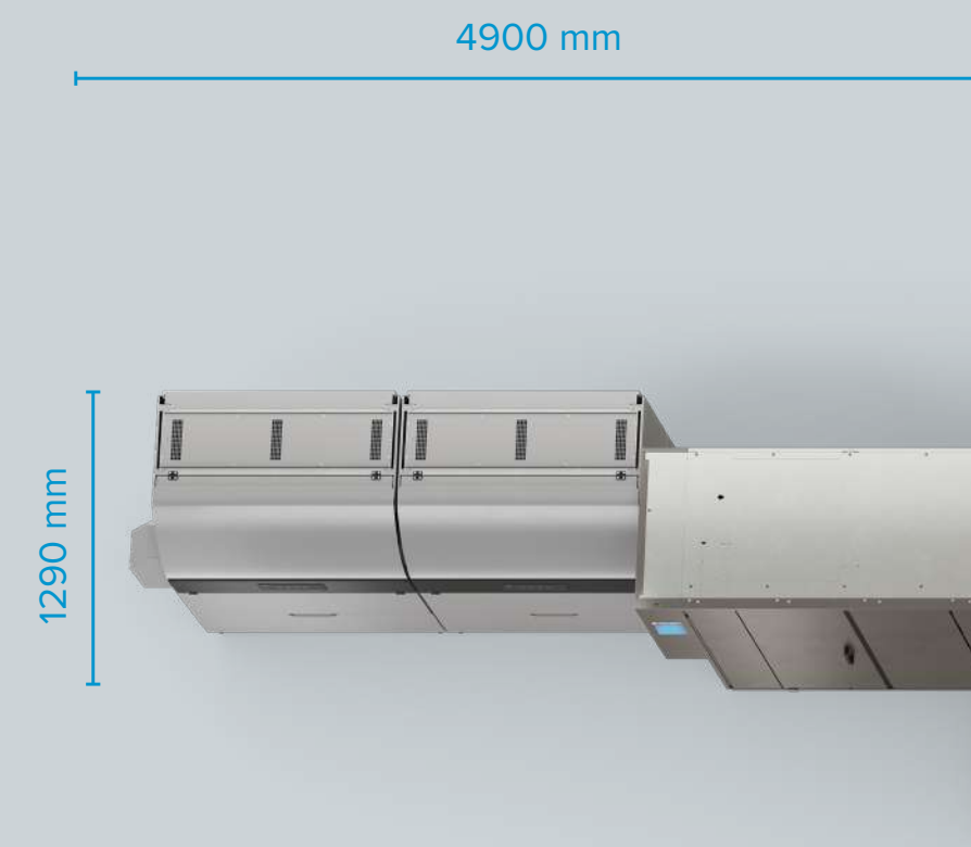
TOMRA R2 z dwoma modułami EasyPac Along i opróżnianiem kosza po lewej stronie
